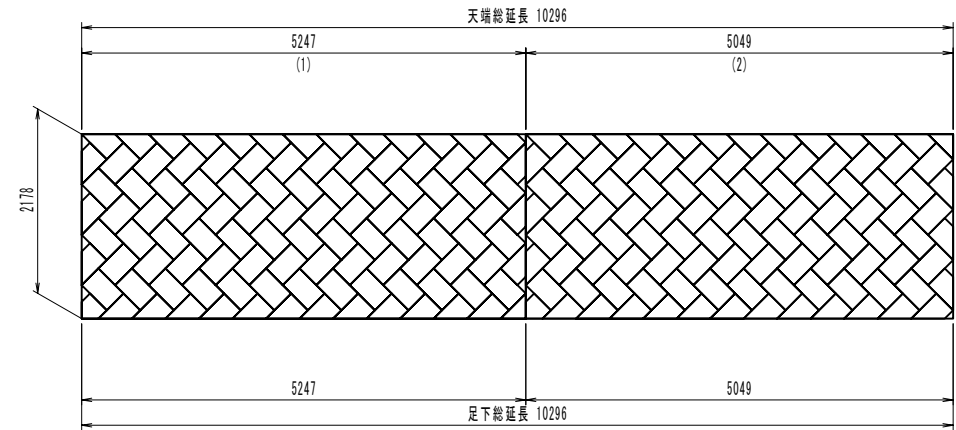
長方形 (特殊根石) s = 1:60
