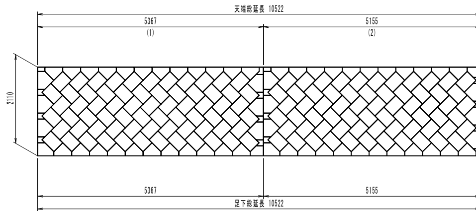
長方形 (M字) s = 1:60
